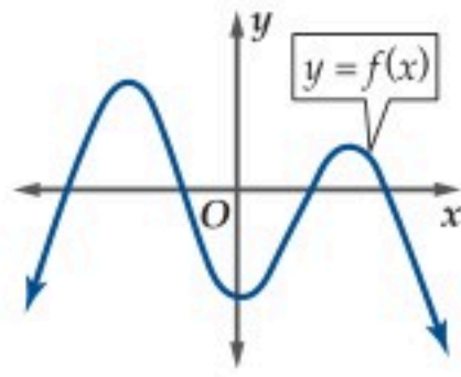
f(x) متصلة لجميع قيم x .
