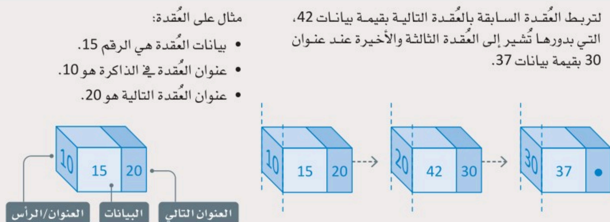
شكل 1.31: المؤشرات في القائمة المترابطة
