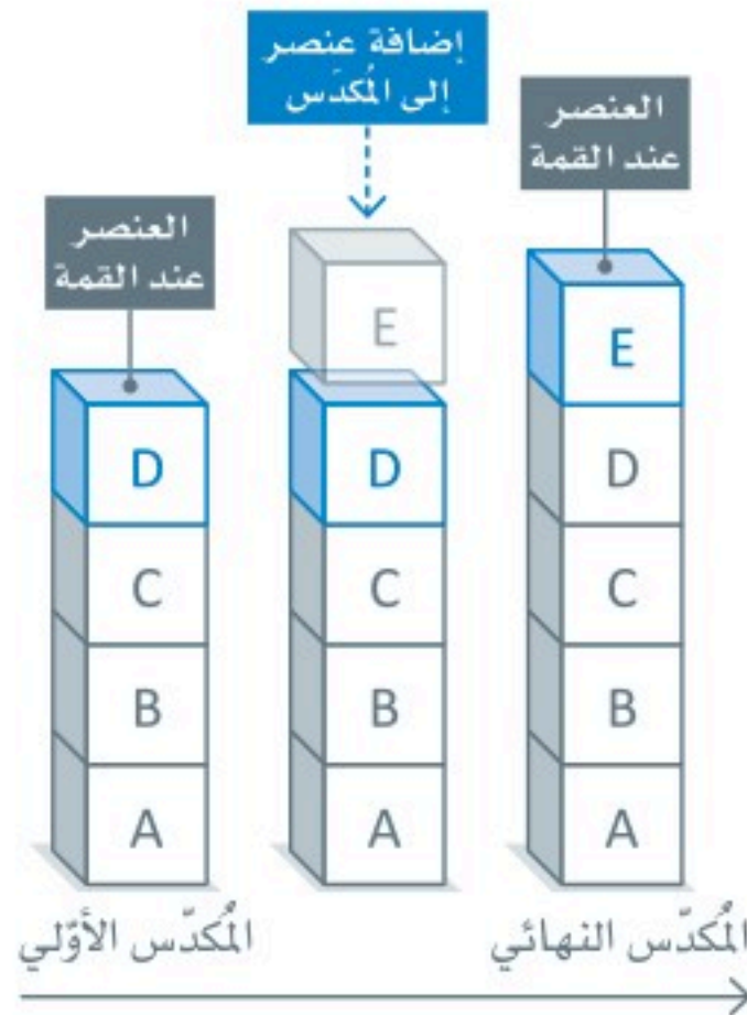
شكل 1.13: عملية إضافة عنصر إلى المُكدّس
