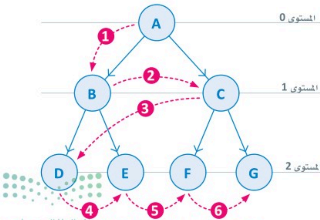
شكل 2.6: خوارزمية البحث بأولوية الاتساع (BFS)
