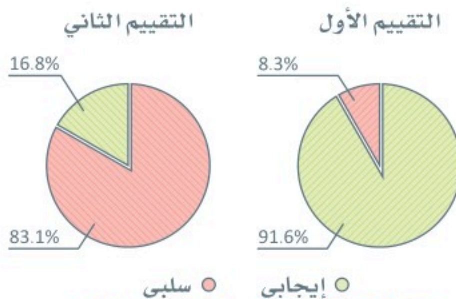
شكل 3.7: مخططان دائريان يوضحان النسب المئوية للتقييمين
