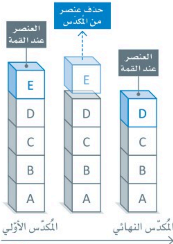
شكل 1.14: عملية حذف عنصر من المُكدّس
