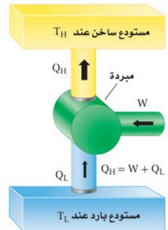
■ الشكل 6-13 يمتص المبرد الحرارة Q_L من المستودع البارد ويبيع الحرارة Q_H إلى المستودع الساخن، ببذل شغل W على المبرد.
