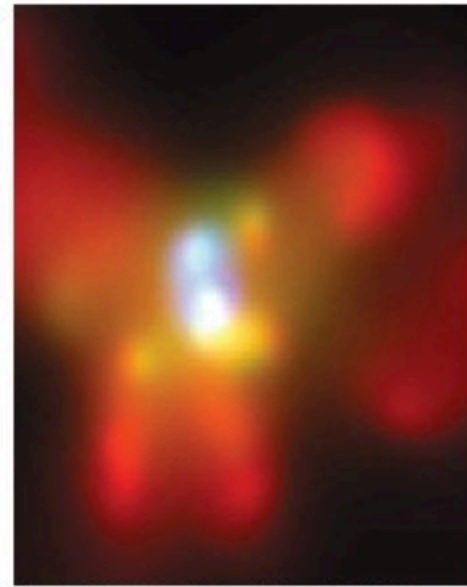
صورة شاندرا بالأشعة السينية للثقبين أسودين في NGC 6240.
