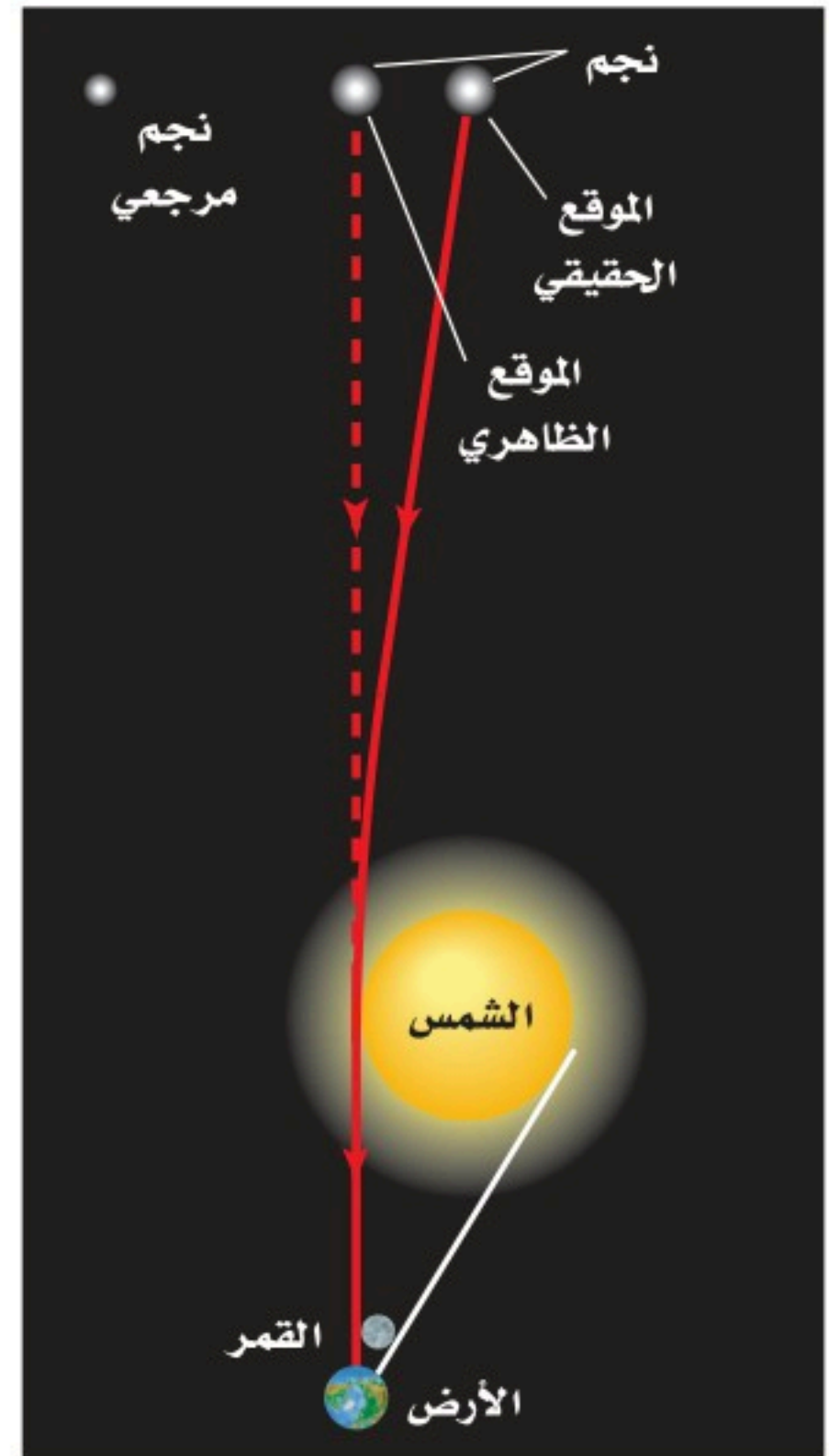
■ الشكل 17-1 الضوء القادم من النجوم البعيدة يتأثر بمجال جاذبية الشمس. الرسم للتوضيح ولا يمثل مقياس رسم حقيقي.
