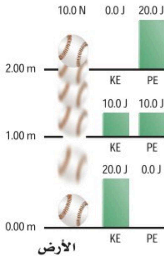
الشكل 5-9: الانقص في طاقة الوضع يساوي الزيادة في الطاقة الحركية.
