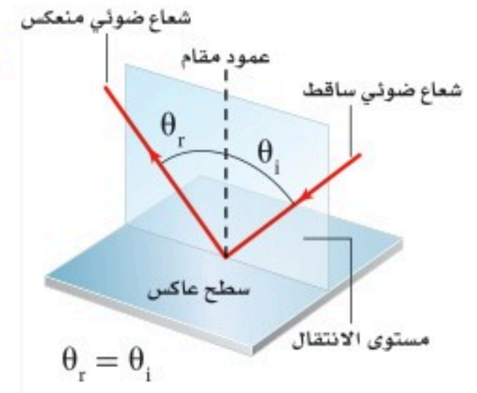
■ الشكل 5-1 يقع كل من الشعاع الساقط والشعاع المنعكس ضمن مستوى الانتقال نفسه.
