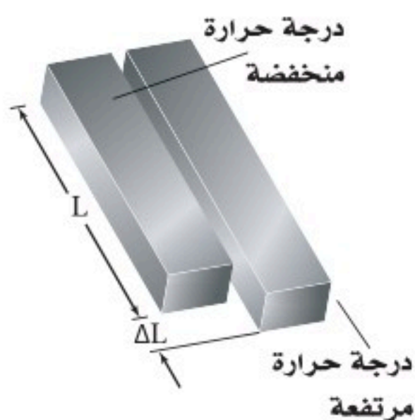
■ الشكل 1-21 يتناسب التغير في طول المادة طردياً مع الطول الأصلي والتغير في درجة الحرارة.
