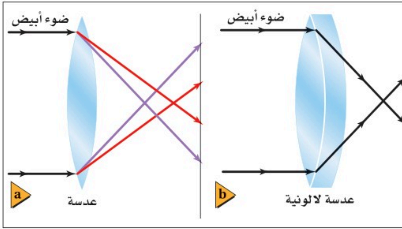
■ الشكل 6-15 للعدسات البسيطة جميعها زوجان لوني، حيث يتركز الضوء ذو الأطوال الموجية المختلفة في نقاط مختلفة (a). العدسة اللالونية نظام من العدسات يؤدي إلى تقليل العيب اللونى (b).
