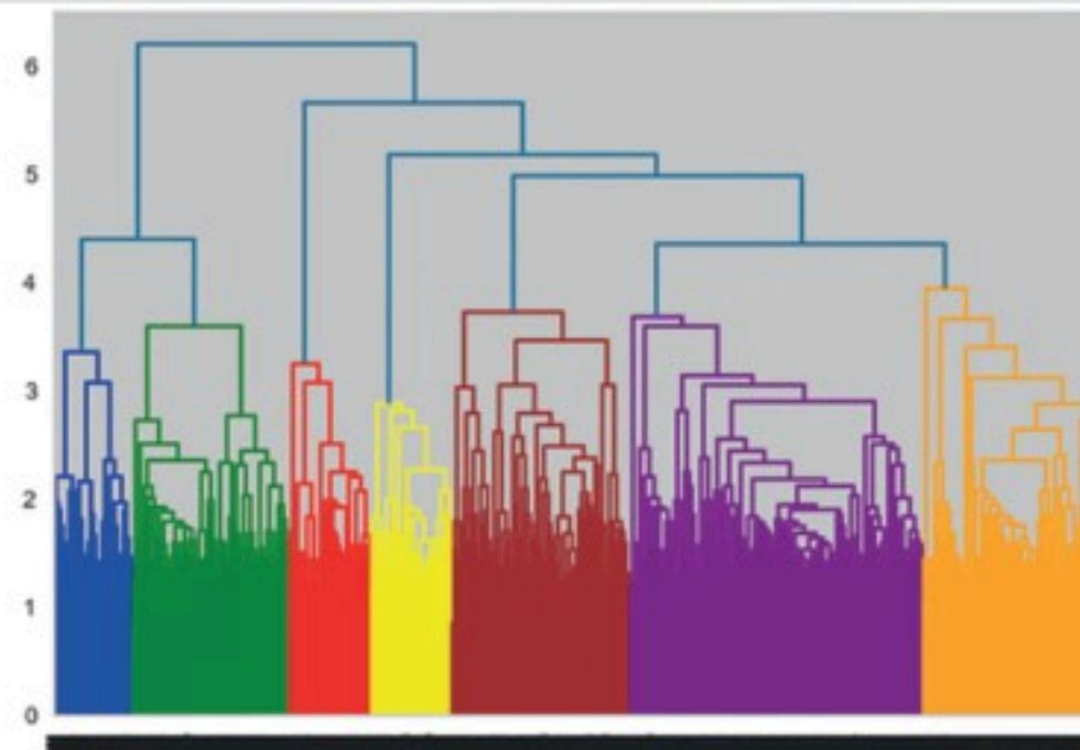
شكل 3.20: الرسم الشجري الهرمي لبيانات هيئة الإذاعة البريطانية
