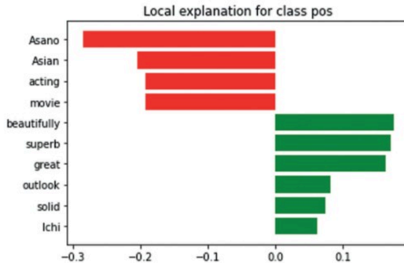
شكل 3.11: الكلمات التي أثرت على القرار الخاطئ
