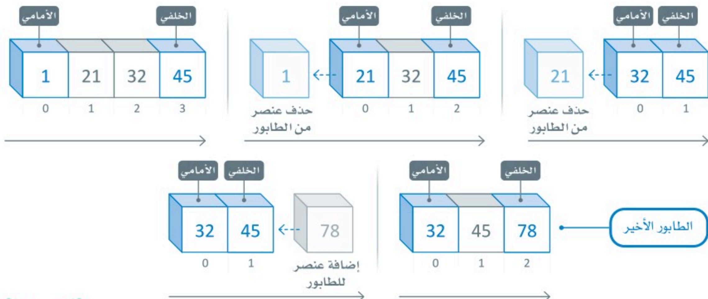
شكل 1.25: مثال توضيحي لفهم الطابور
