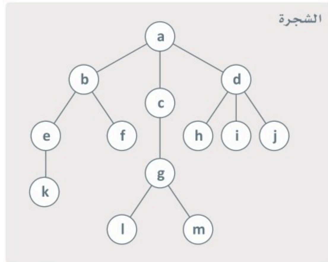
شكل 1.40: الشجرة والشجرة الثنائية
