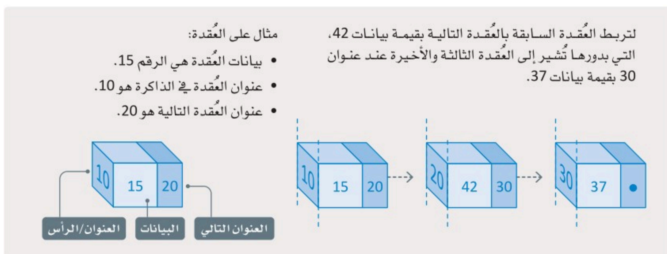
شكل 1.31: المؤشرات في القائمة المترابطة
