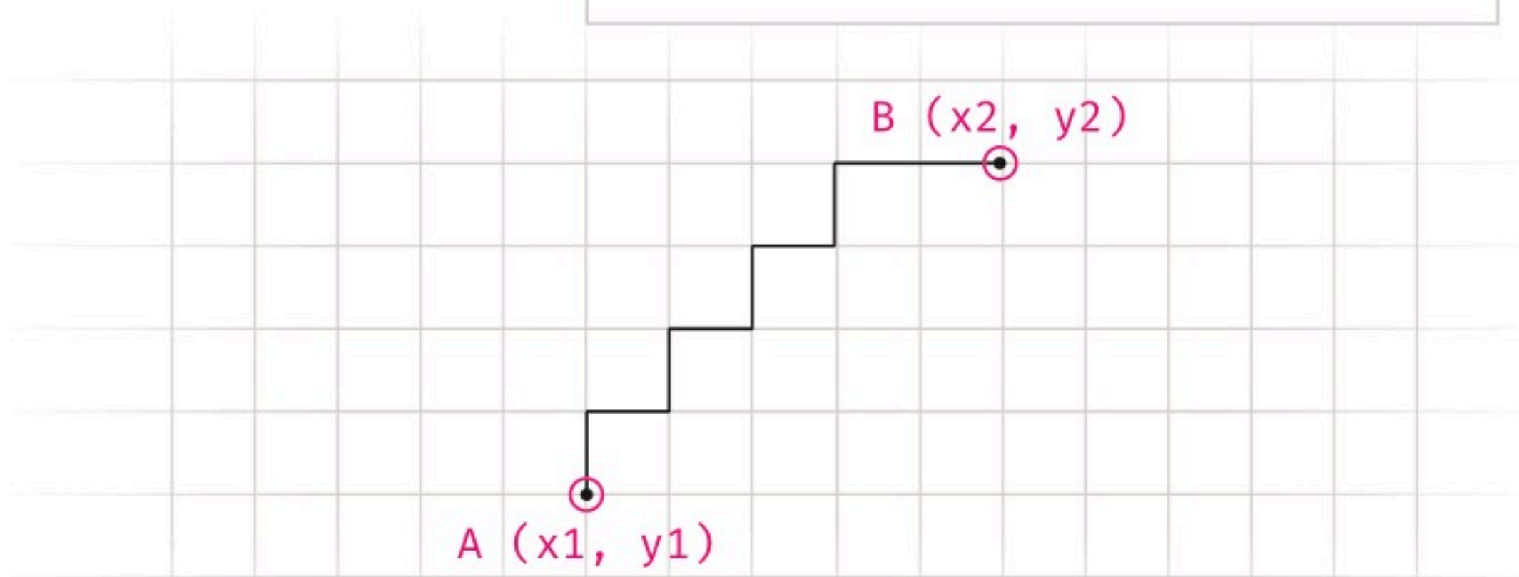
شكل 2.25: مسافة مانهاتن
