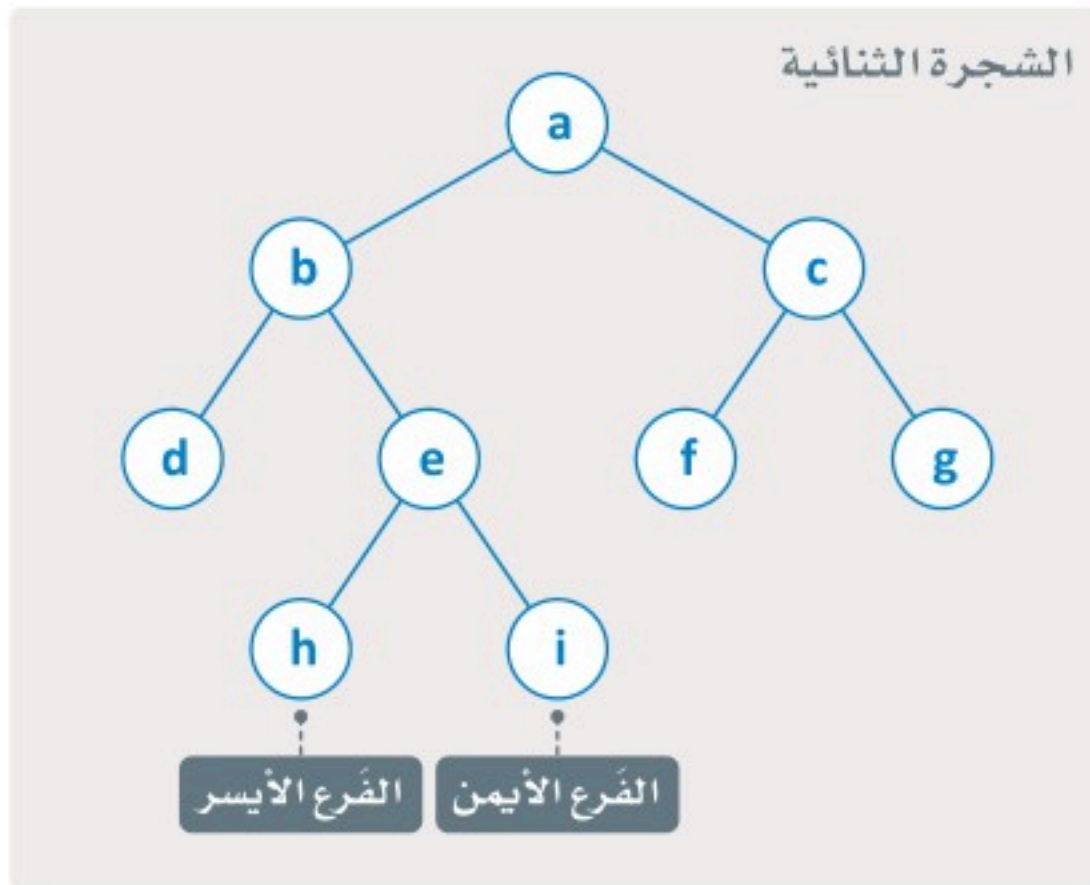
شكل 1.40: الشجرة والشجرة الثنائية
