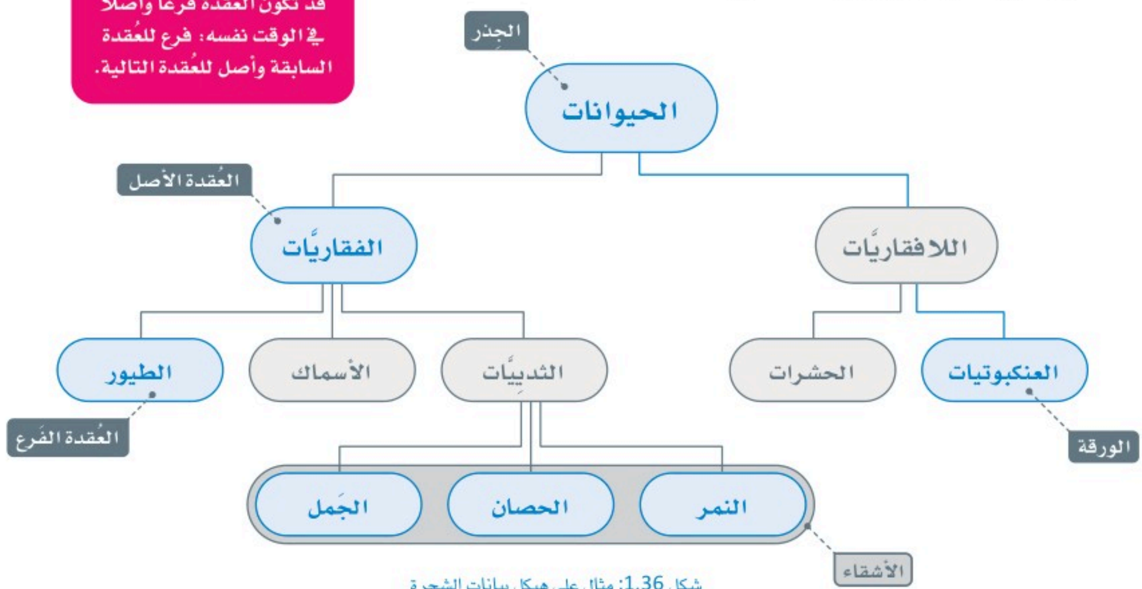
شكل 1.36: مثال على هيكل بيانات الشجرة
