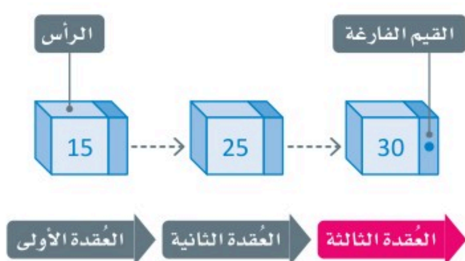
شكل 1.30: الوصول إلى العقدة الثالثة في القائمة المترابطة
