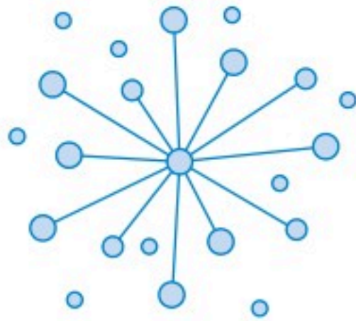
شكل 3.16: تمثيل عنقود
